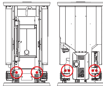
Fig. 9 CANALISATION
